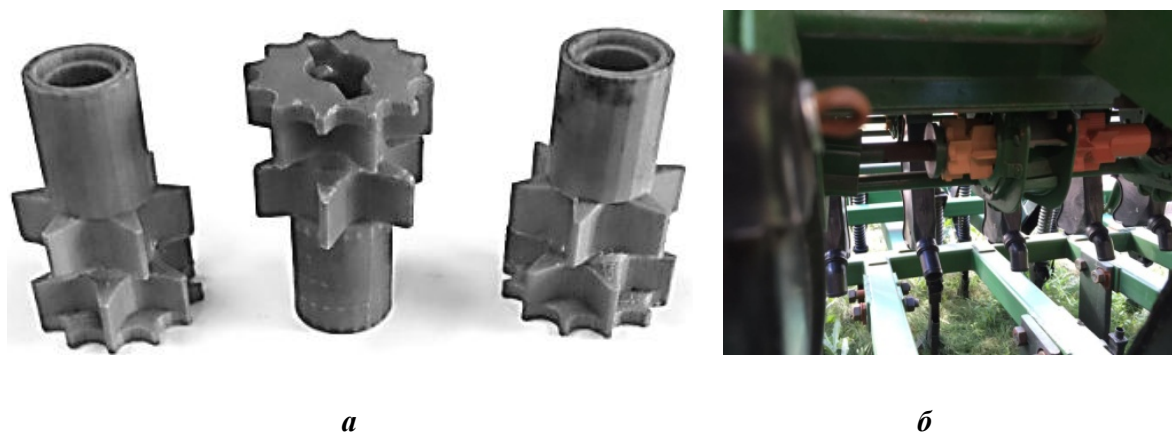
а - изготовленные катушки; б - катушки, установленные в бункере
