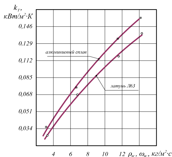
Рисунок 2 – Коэффициент теплопередачи трубчато-пластинчатых радиаторов из ленты латунной Л63 и алюминиевого сплава
