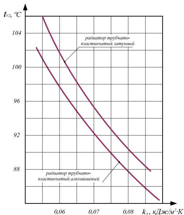
Рисунок 4 – Температура охлаждающей жидкости трактора «БЕЛАРУС-80.1» в зависимости от коэффициента теплопередачи
