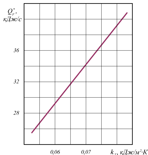
Рисунок 3 – Теплоотдача поверхности охлаждения радиатора трактора «БЕЛАРУС-80.1» в зависимости от коэффициента теплопередачи
