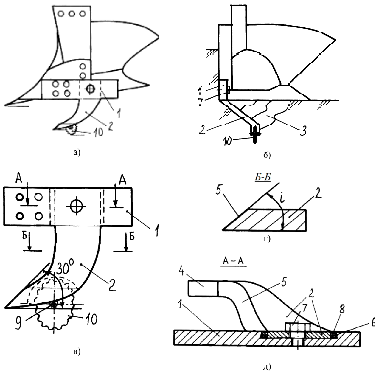
Рисунок 1 – Плуг-удобритель
