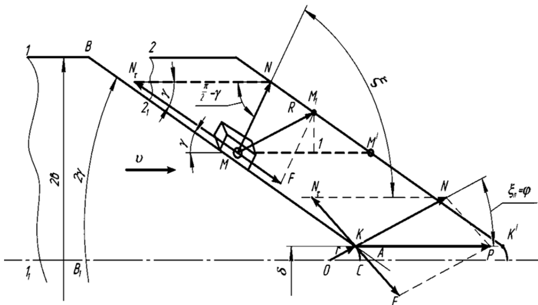
Рисунок 3 - К обоснованию параметров сошника-щелевателя
