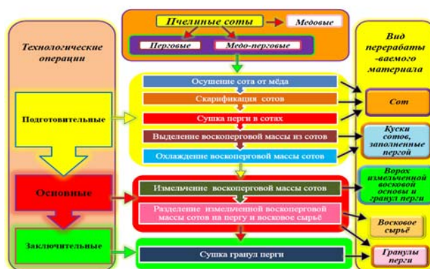
Рис. 1 – Схема технологического процесса промышленной переработки пчелиных сотов на пергу и восковое сырьё.
