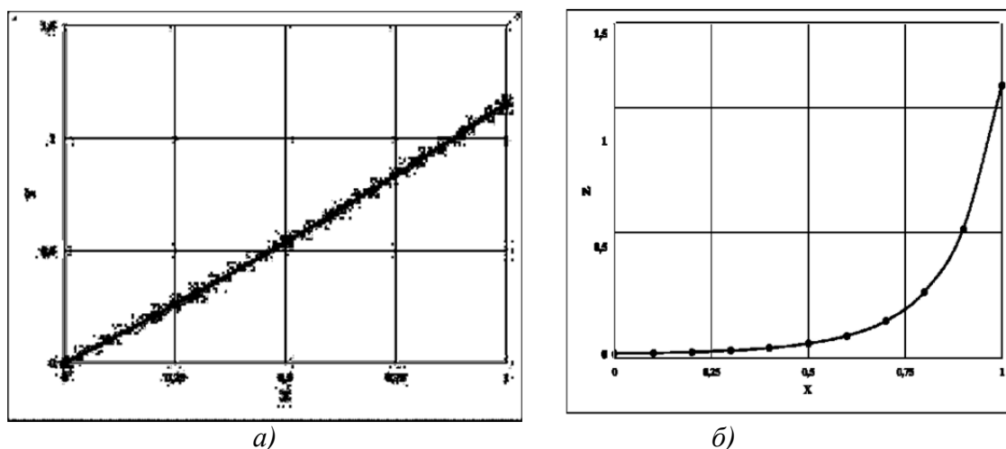
а-проекции траектории движения частицы на плоскости XOY ; б-проекции траектории движения частицы на плоскости XOZ
