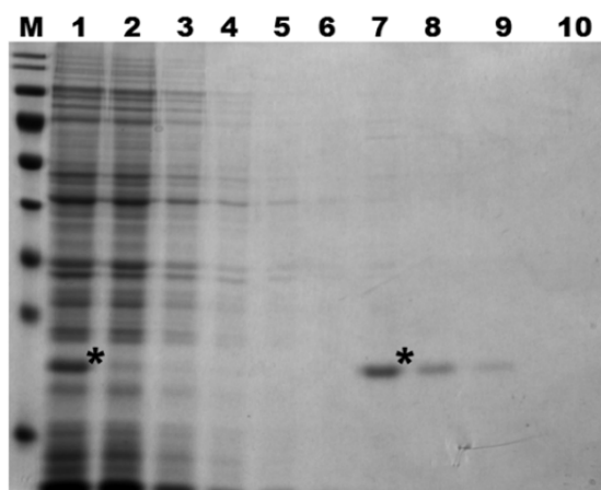
М – маркер молекулярного веса; 1 – общий клеточный лизат; 2 – проток через колонку; 3-6 – отмывка; 7-10 – элюция белка (рекомбинантный белок Omp25 обозначен звездочкой.)
