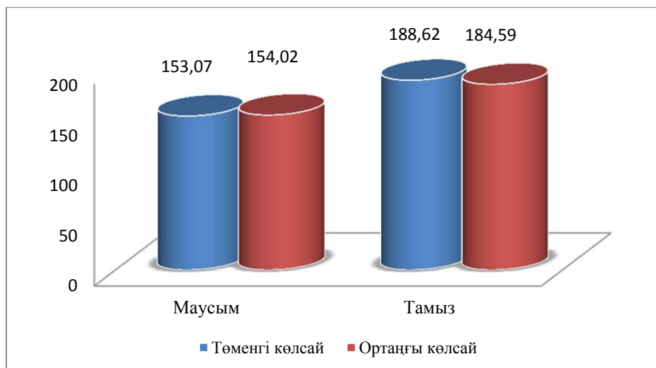
Сурет 3–Ортаңғы Көлсай және Төменгі Көлсай көлдерінің 2019 жылғы зерттеу кезеңдеріндегі минералдану көрсеткіштері
