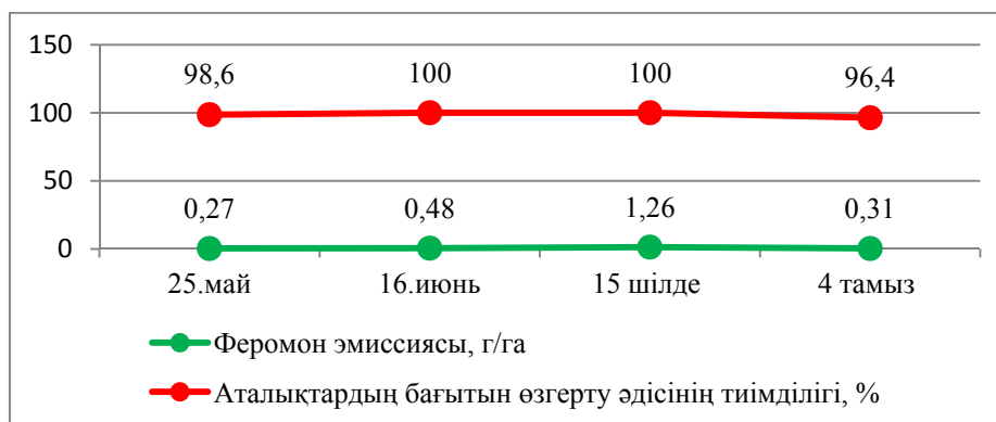
Сурет 1 – Алматы облысы, Еңбекшіқазақ ауданы, «Жеміс» шаруа қожалығы дизрапторларындағы феромон эмиссиясының динамикасы (г) және аталықтардың бағытын өзгерту әдісінің тиімділігі (%), (2016 ж.).
