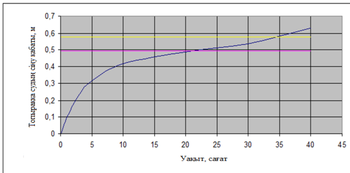
Сурет 1. Тамшылатып суғарғанда топыраққа судың сіну қисығы.
