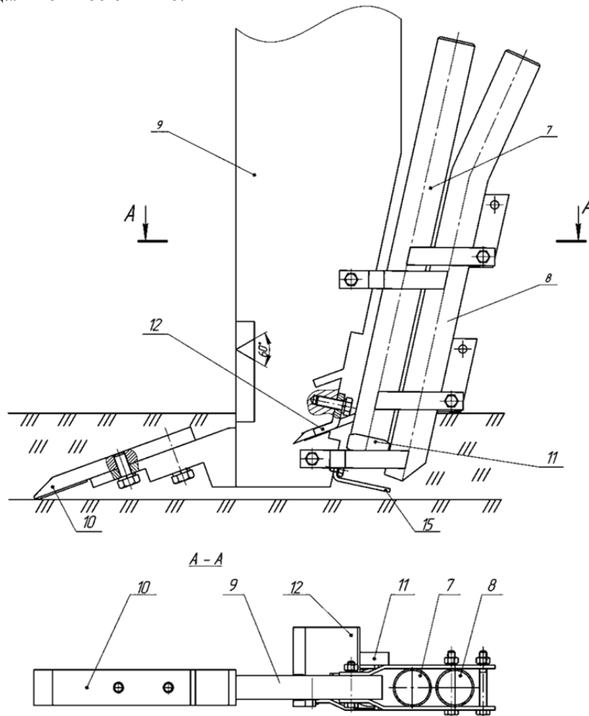
Рисунок 2 - Экспериментальный сошник-щелеватель
